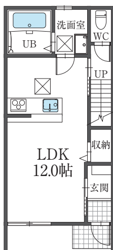
A棟 平面図
