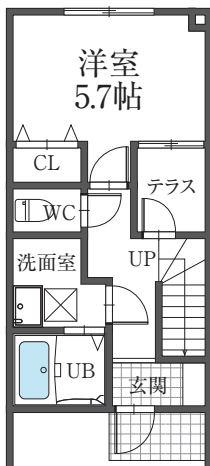
1階 平面図
