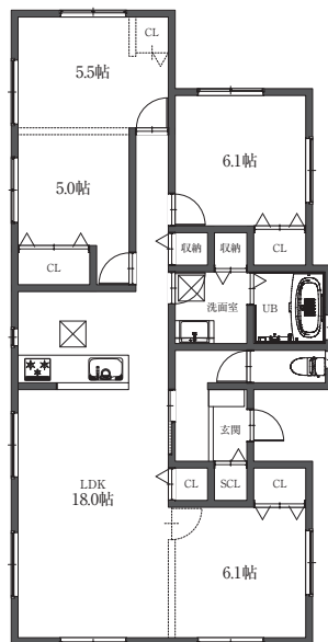
B棟 平面図
