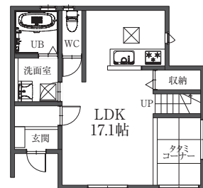
B2棟 1階 平面図
