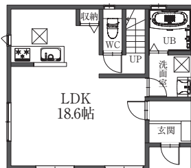
B1棟 1階 平面図
