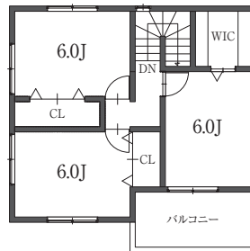
B1棟 2階 平面図
