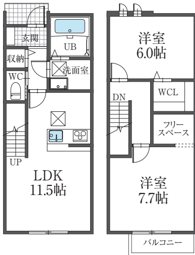
A棟 平面図
