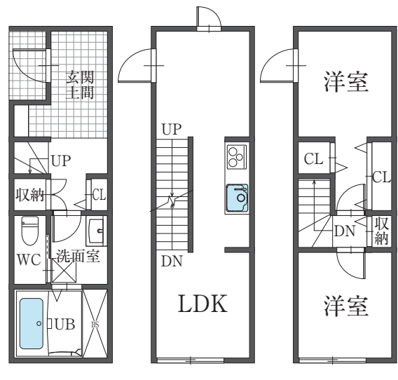
105号 平面図
