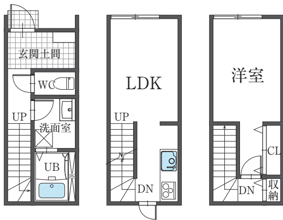
101~103号 平面図
