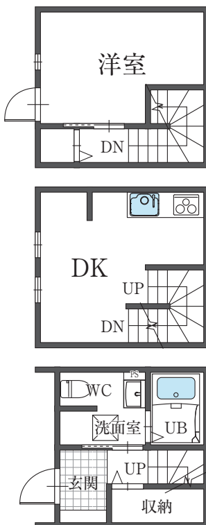
Atype 平面図
