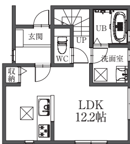
A棟 1階 平面図
