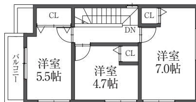
B棟 2階 平面図
