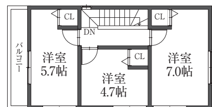
C棟 2階 平面図
