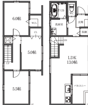
B1 平面図
