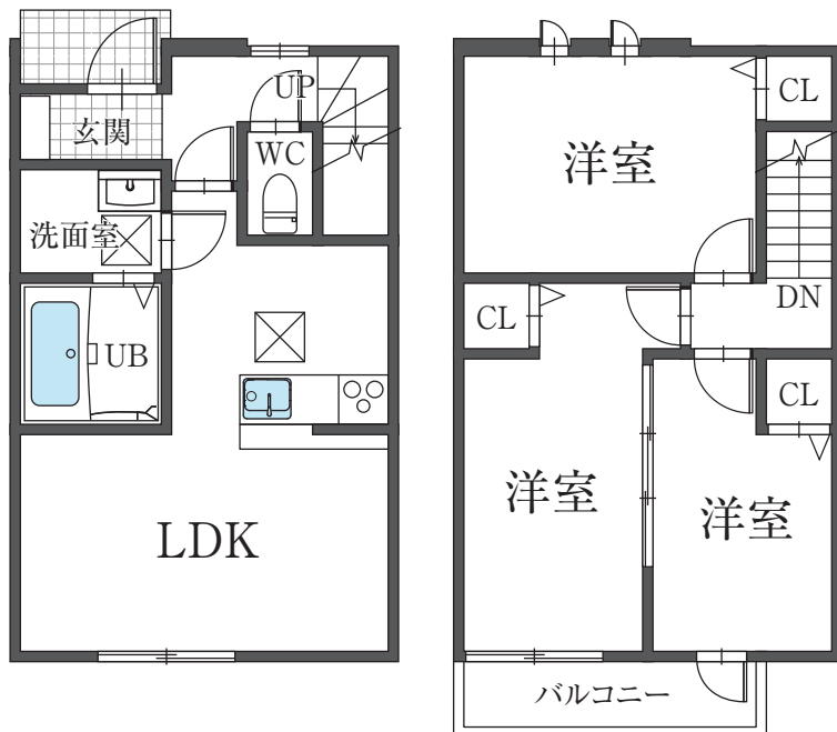
101号 平面図
