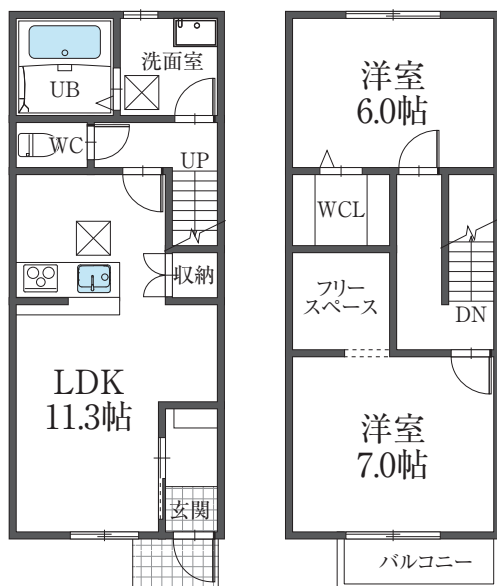
平面図
