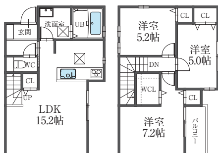
A棟 平面図
