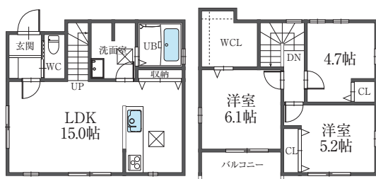
C棟 平面図
