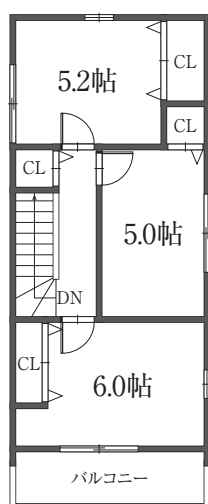
A棟 平面図
