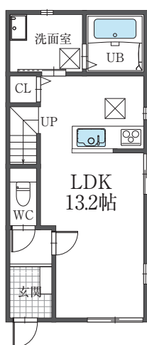
A棟 平面図
