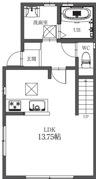
1F 平面図
