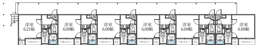
1階 平面図
