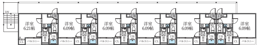
3階 平面図
