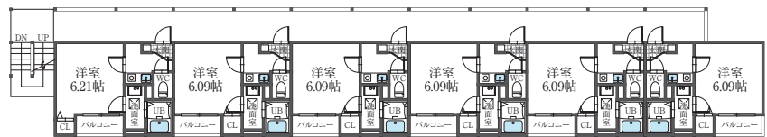
2階 平面図
