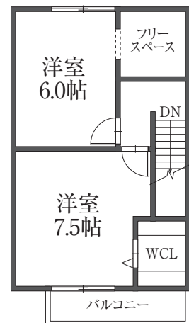
B棟平面図
