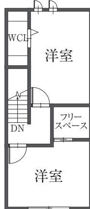
B棟 平面図
