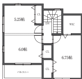
C棟 平面図
