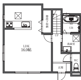
C棟 平面図
