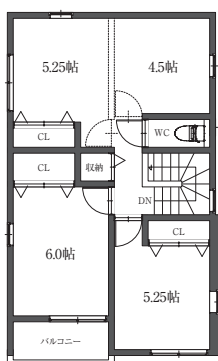
A棟 平面図
