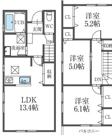
E棟 平面図
