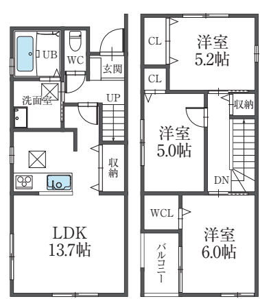
F棟 平面図
