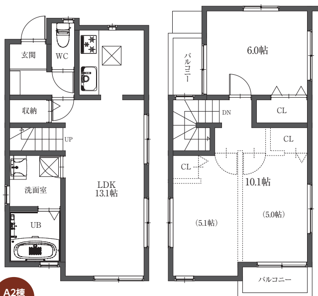
A2棟 平面図
