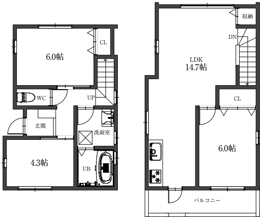
C棟 平面図
