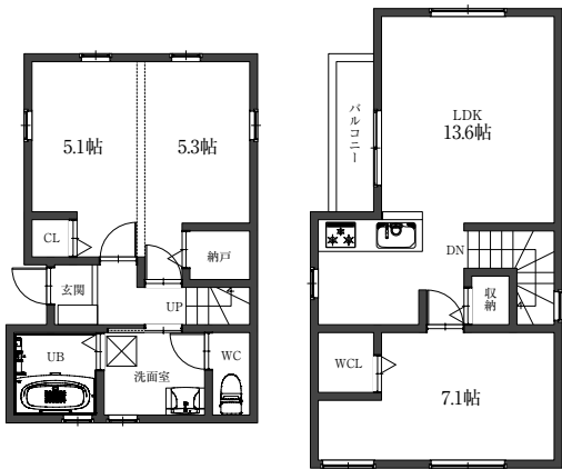
A棟 平面図
