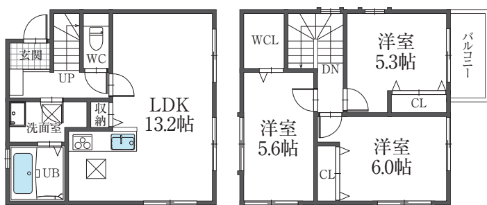
A・B棟 平面図
