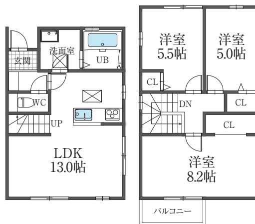
D棟 平面図
