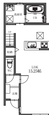
B2棟 平面図
