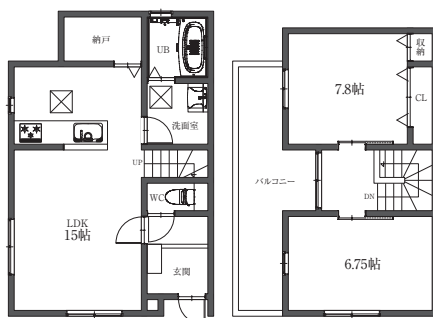
B1棟 平面図
