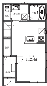
B1 平面図
