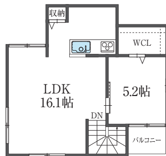
A棟 平面図
