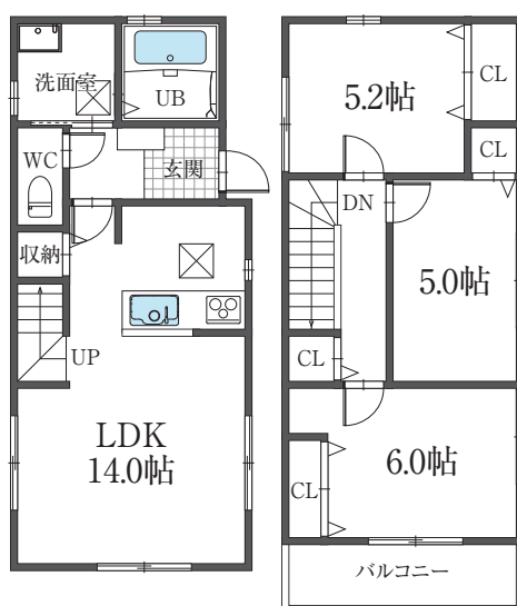
C棟 平面図
