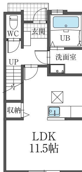
A棟1階 平面図
