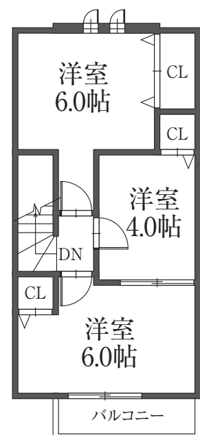
A棟2階 平面図
