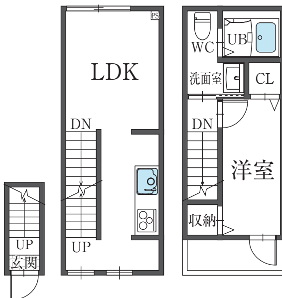
201号 平面図
