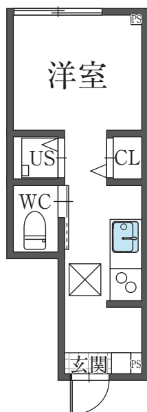
101号 平面図
