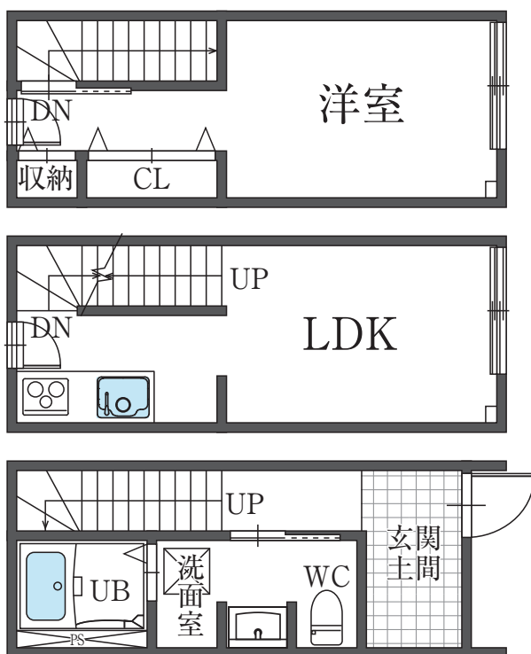
102号 平面図
