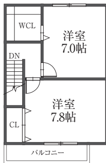
A棟 平面図
