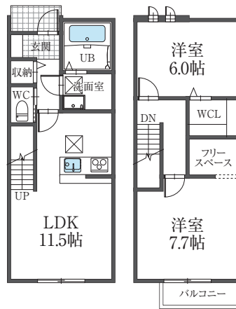
B棟 平面図
