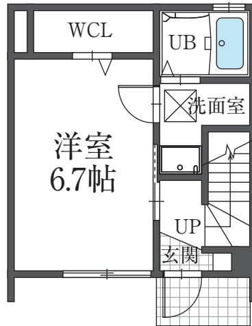
1階 平面図
