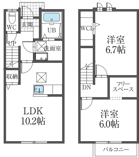
1階 平面図
