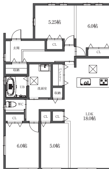
B棟 平面図
