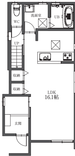
D棟 平面図
