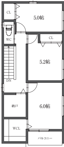
A棟 平面図
