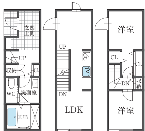
105号 平面図
