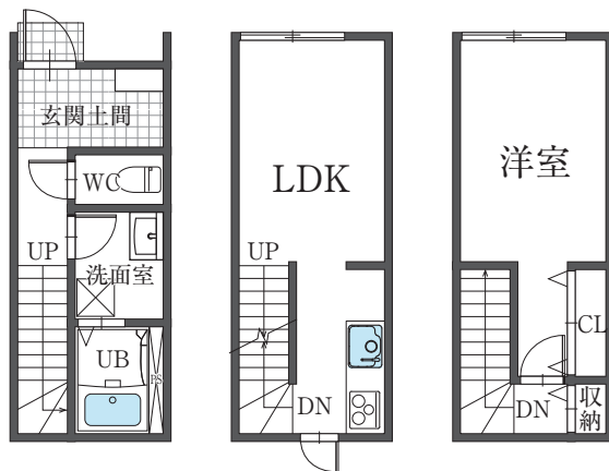
101～103号 平面図
