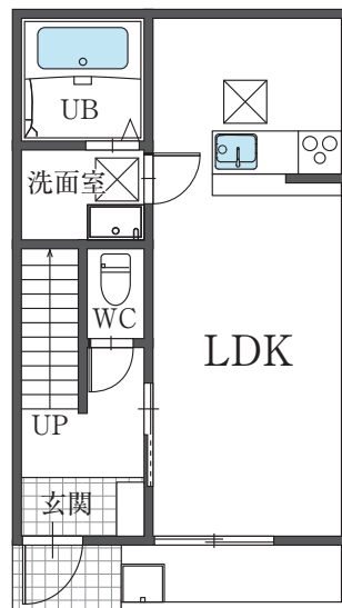
1階 平面図
