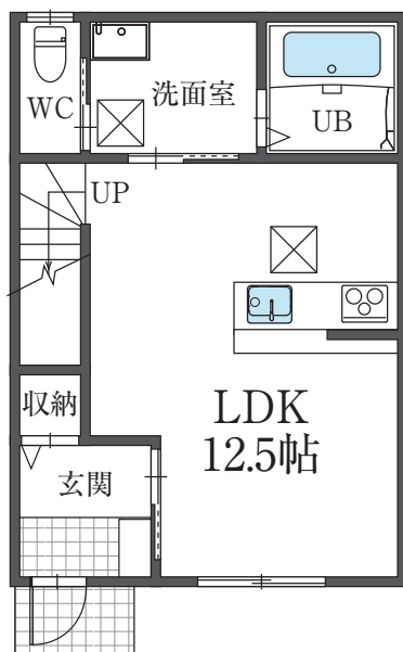
B棟101号 平面図
