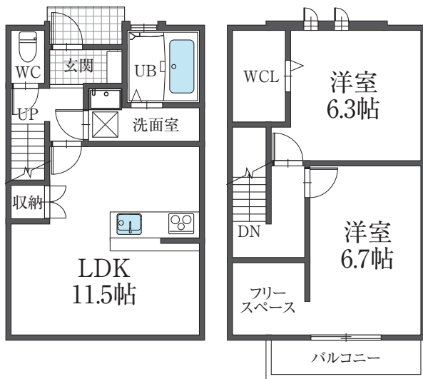
C棟 平面図
