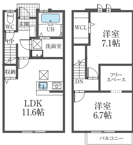
A棟 平面図
