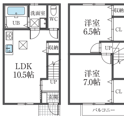
B棟 平面図
