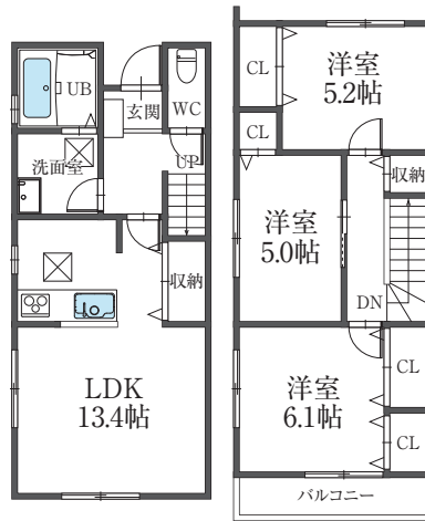
B棟 平面図
