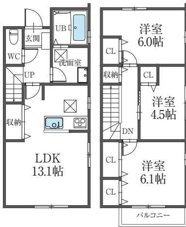
A棟 平面図
