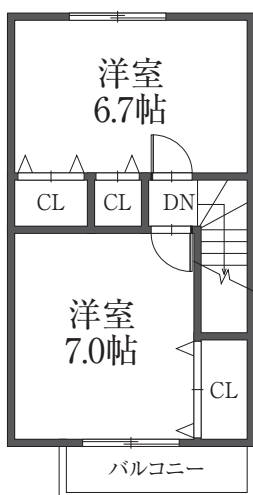
A棟平面図
