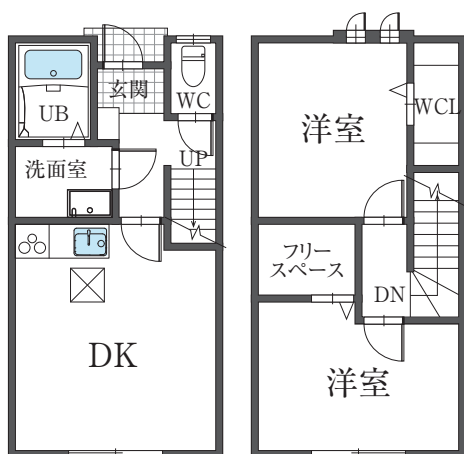
C棟 平面図
