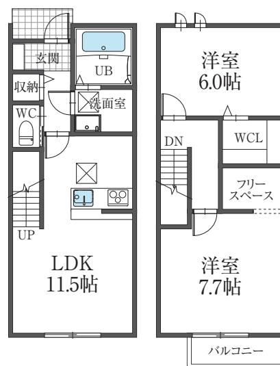
102号 平面図
