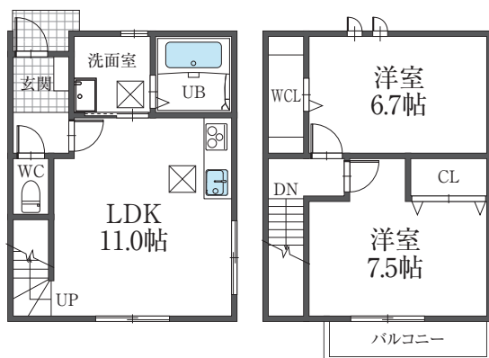
101号 平面図
