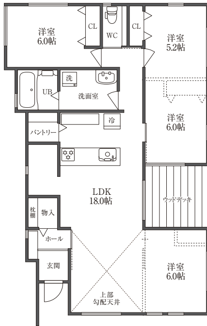
平面図
