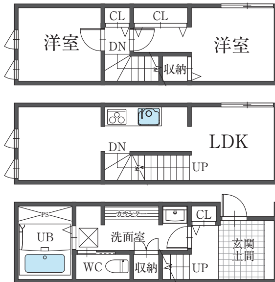
101号 平面図
