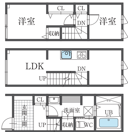
Atype 平面図
