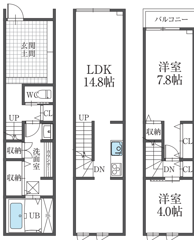
101号 平面図
