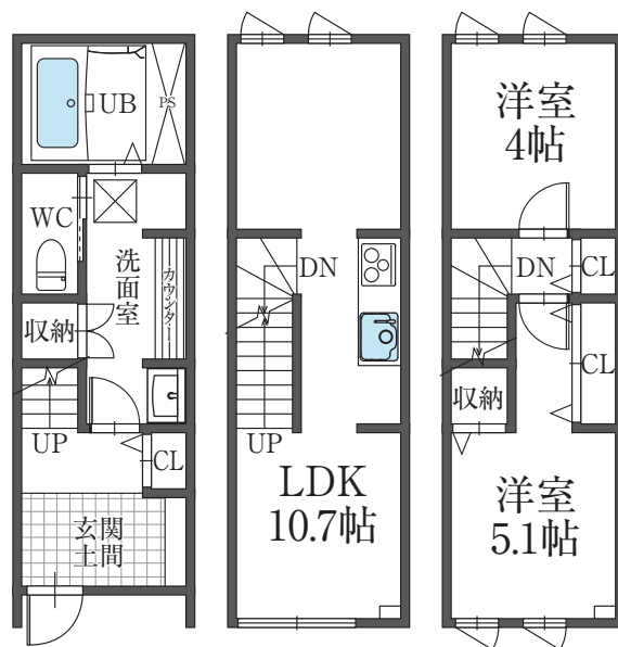
103号 平面図
